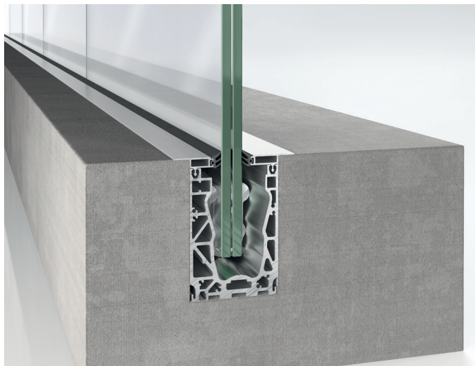
Installazione con incasso a pavimento
