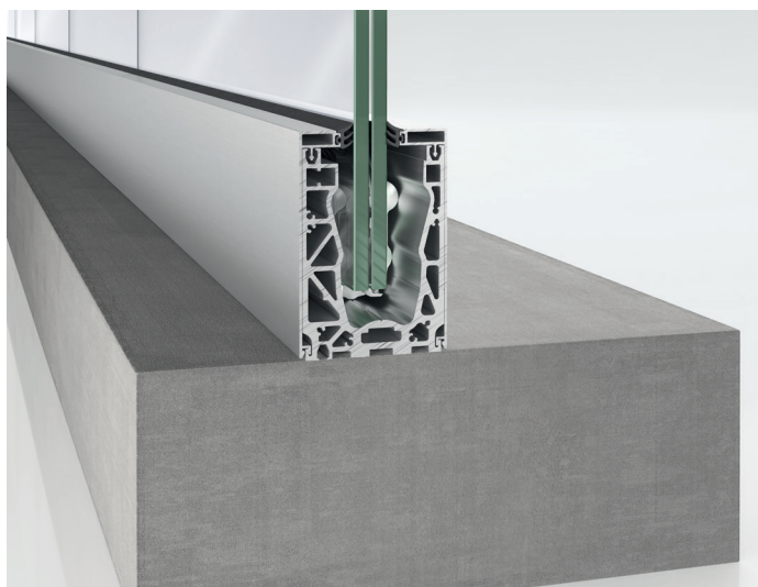
Installazione a pavimento
