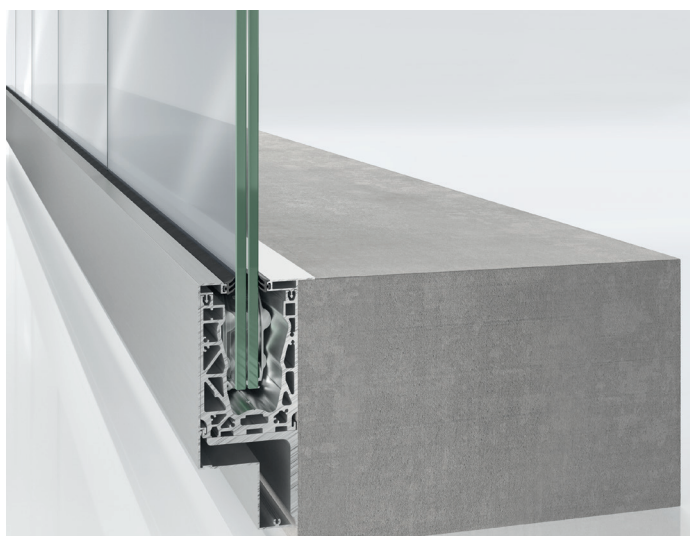
Installazione fronte soletta
